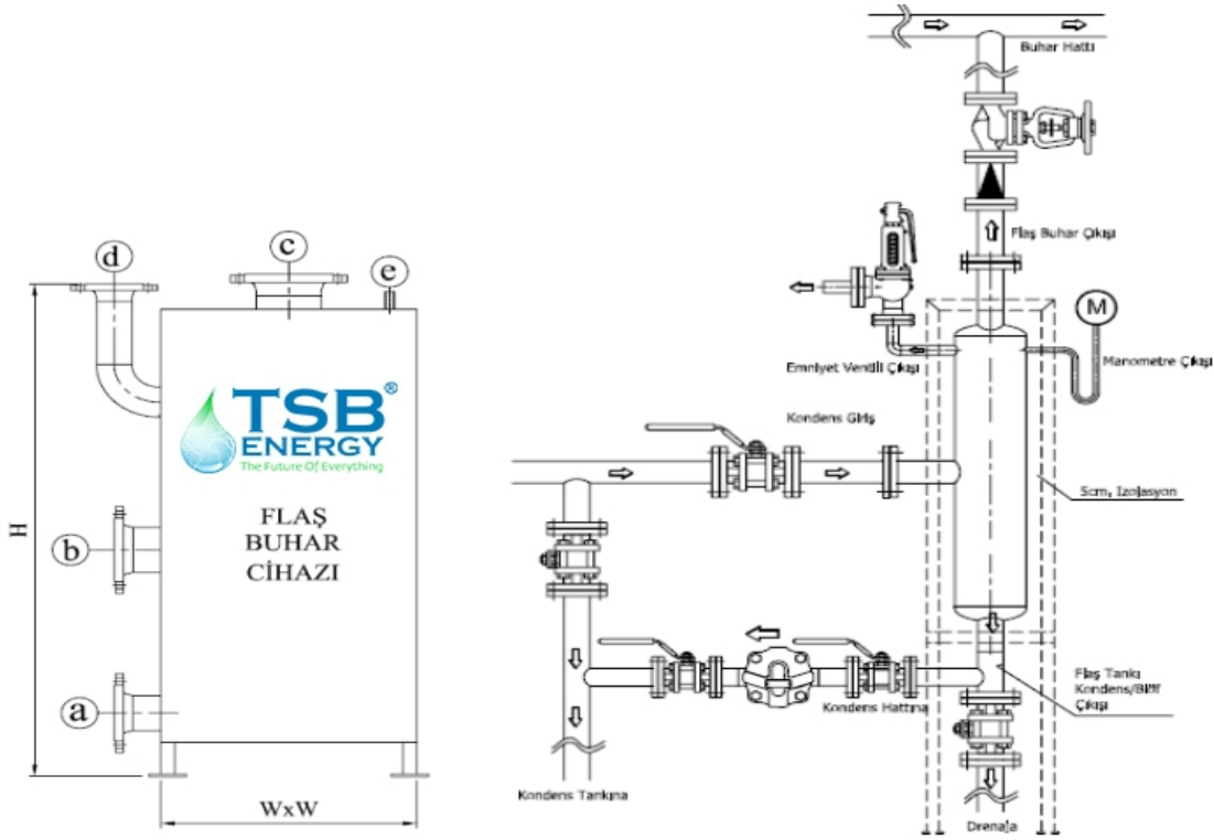
Flaş buhar cihazı bağlantı şeması.
